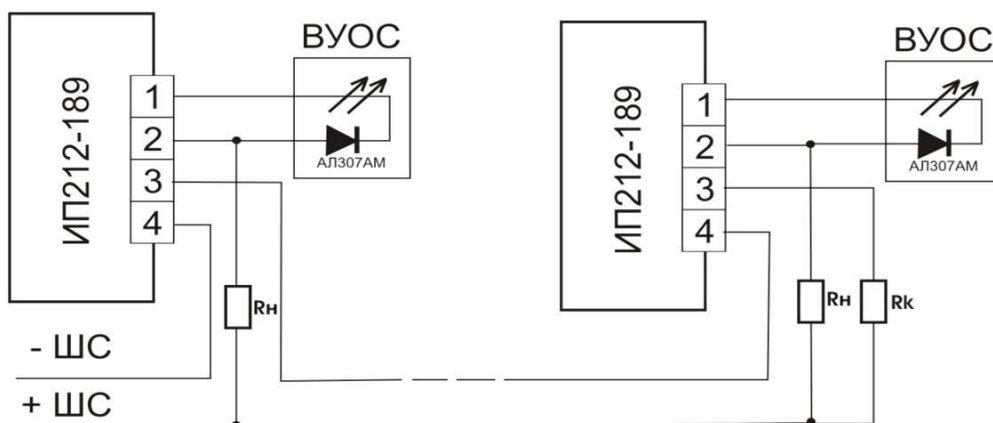
Рис 1. Схема подключения извещателей ИП 212-189 «Шмель» к ППКОП производства ЗАО НВП «Болид»
